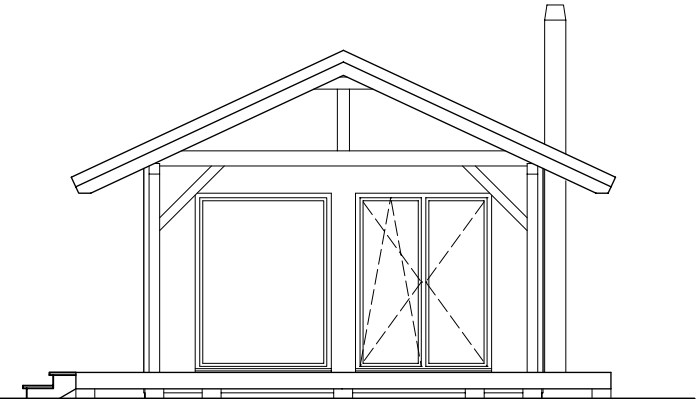
Elewacja boczna prawa
