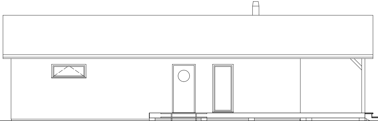
Elewacja frontowa
