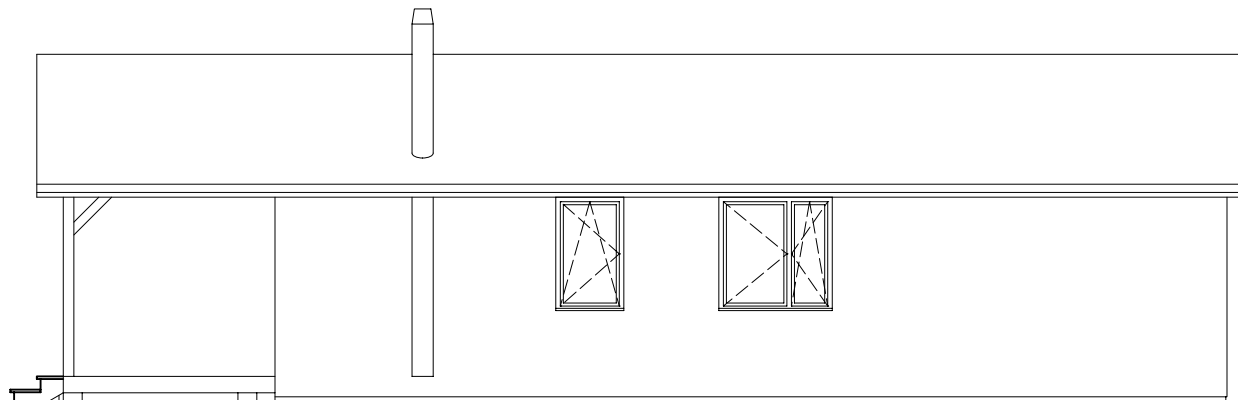
Elewacja tylna
